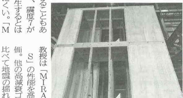
家の模型を用いた振動台実験
